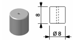
Sellador
