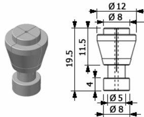
Pinza
