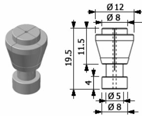
Pinza
