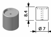
Preguía
