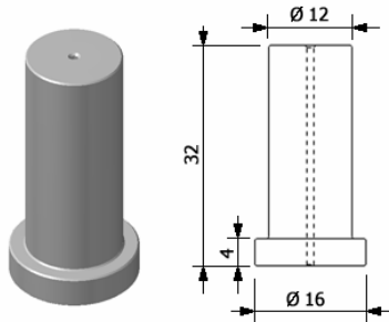
Guía
