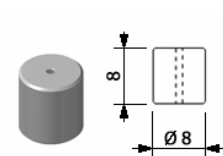
Sellador
